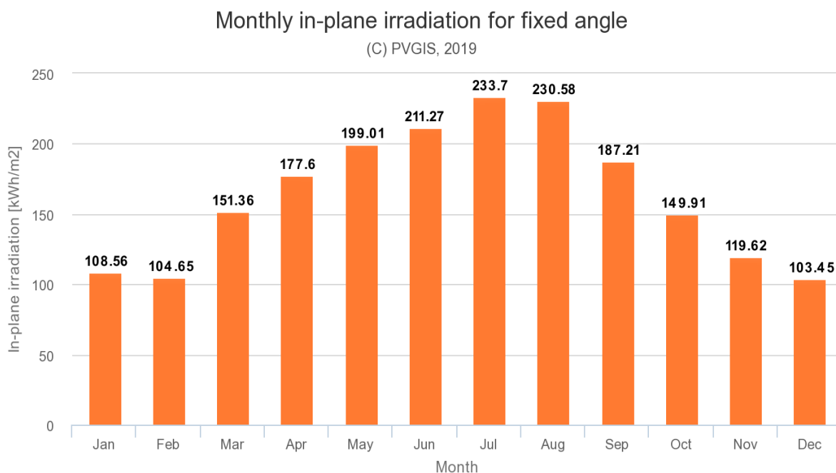
Σχήμα 4-1: Προσπίπτουσα ηλιακή ενέργεια ανά μήνα (Πηγή PVGIS)
