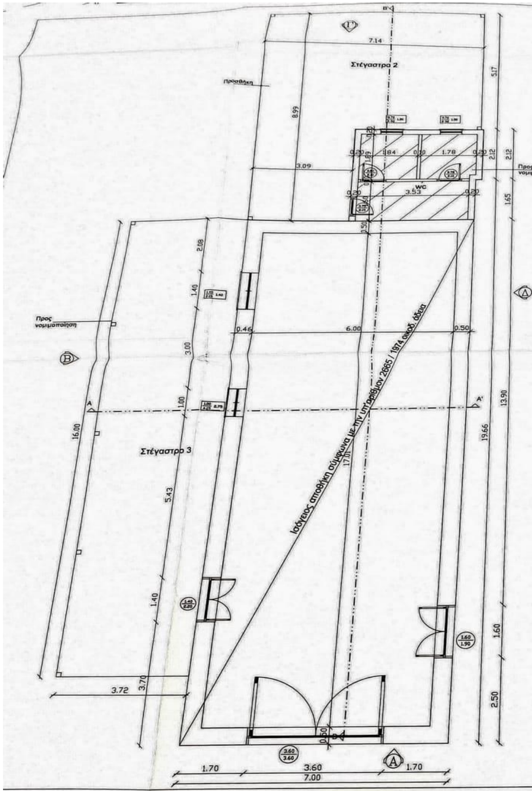
Εικόνα 2-6: Κάτοψη Οινοποιείου
