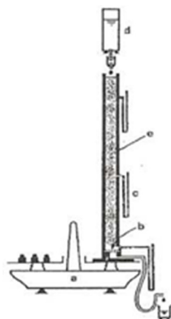
Σχήμα 4. 3: Σχηματική παράσταση στήλης με διάφραγμα πίεσης
