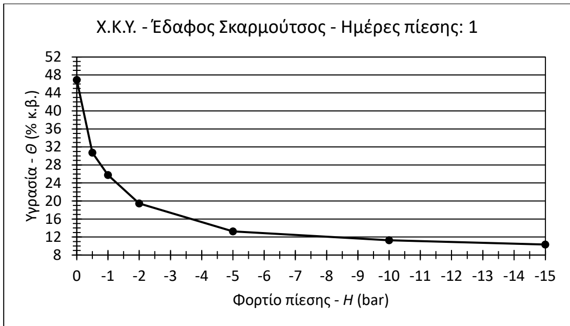
Σχήμα 6. 16: Χαρακτηριστική καμπύλη υγρασίας κατά βάρος, για το δείγμα Σκαρμούτσος μετά από μία ημέρα πίεση
