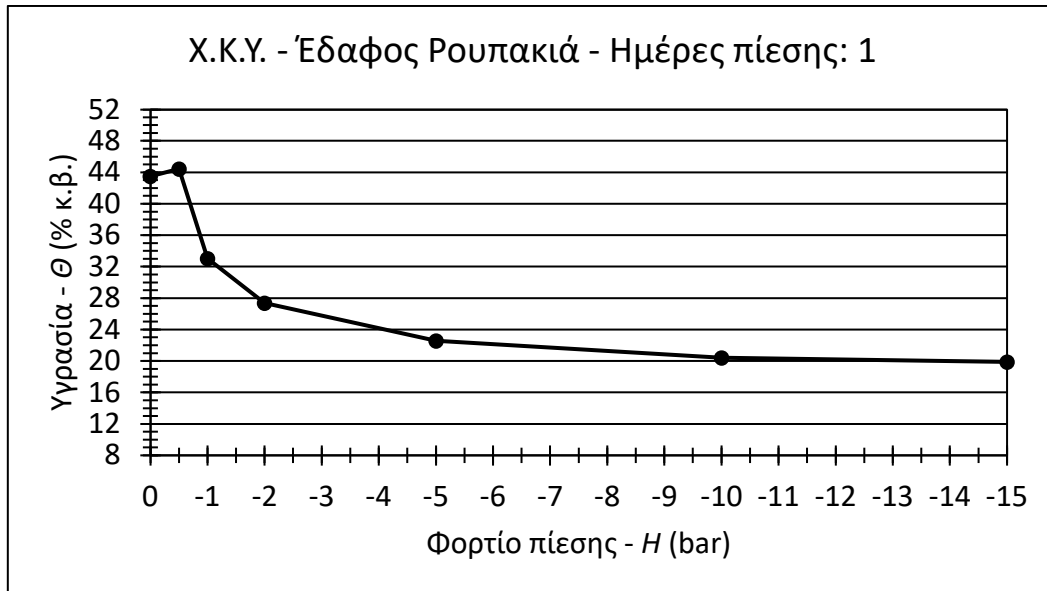
Σχήμα 6. 11: Χαρακτηριστική καμπύλη υγρασίας κατά βάρος, για το δείγμα Ρουπακιά μετά από μία ημέρα πίεσης
