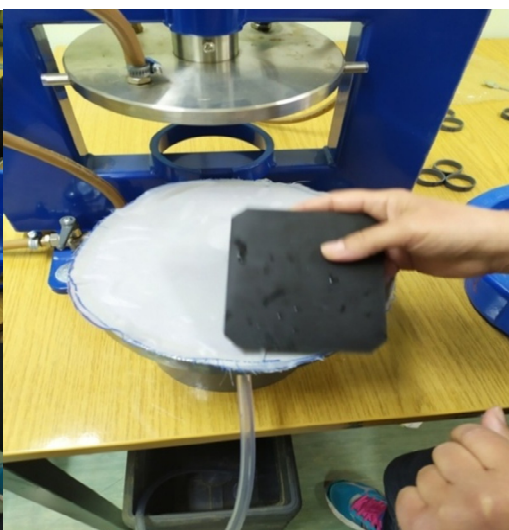
Εικόνα 5.24: Τα 2 φύλλα υφάσματος τοποθετούνται και αφαιρούνται οι φυσαλίδες αέρα.
