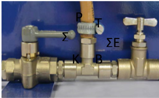
Εικόνα 5.31: Βαλβίδα Α κλειστή και η βαλβίδα Β ανοίγει αργά
