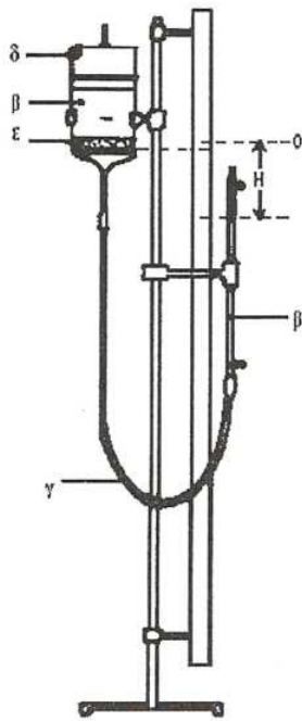
Σχήμα 4. 1: Συσκευή Haines
