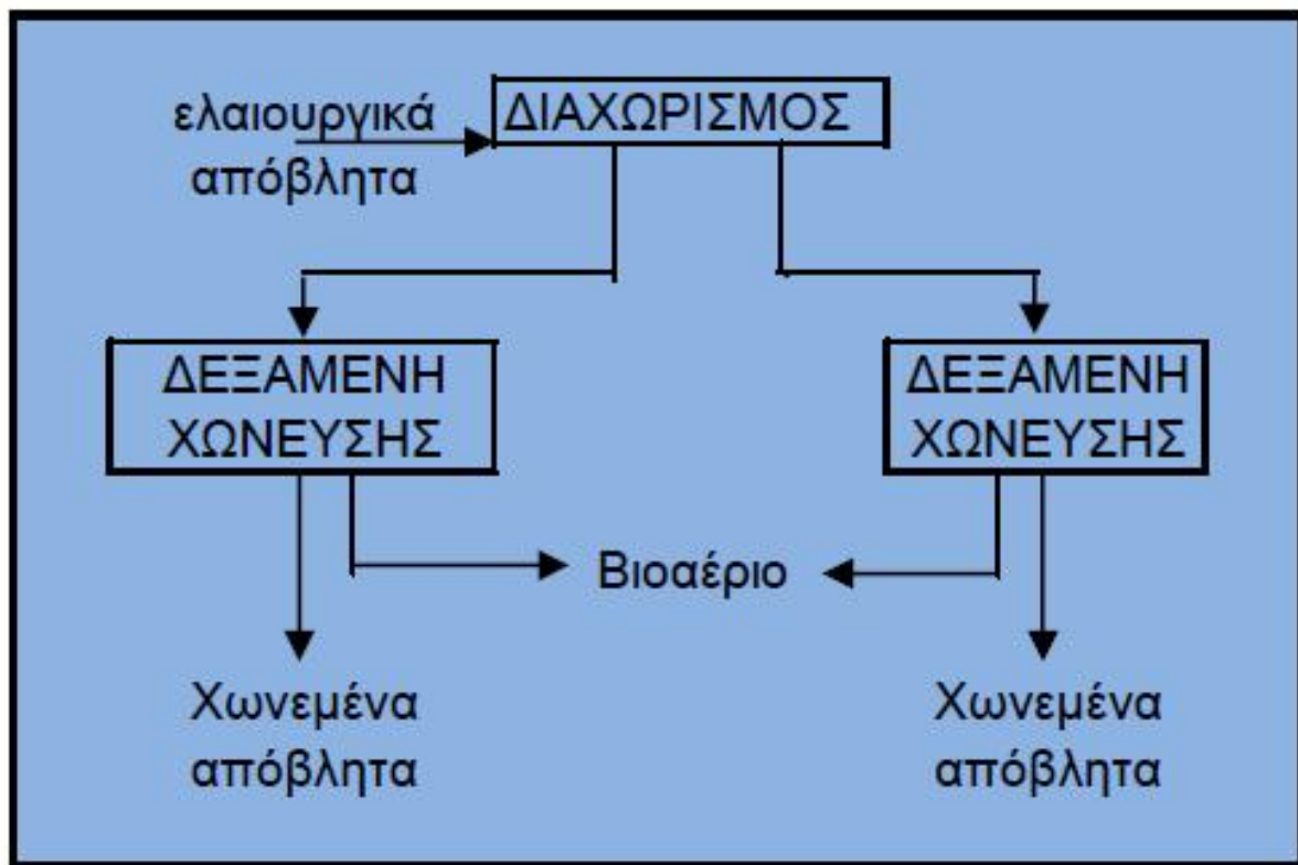
Εικόνα 50: Παραγωγή βιοαερίου από απόβλητα ελαιουργείου.[23]
