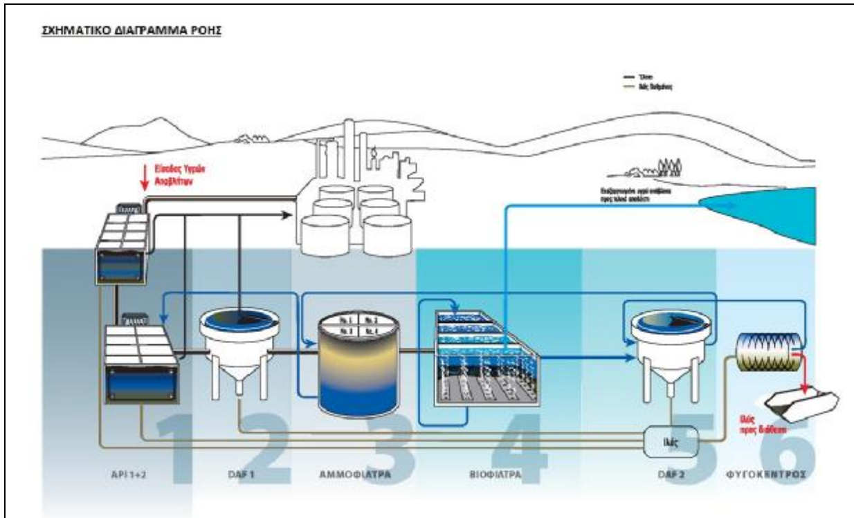
Εικόνα 49: Παραγωγή βιοαερίου από την καθίζηση της ίλως
