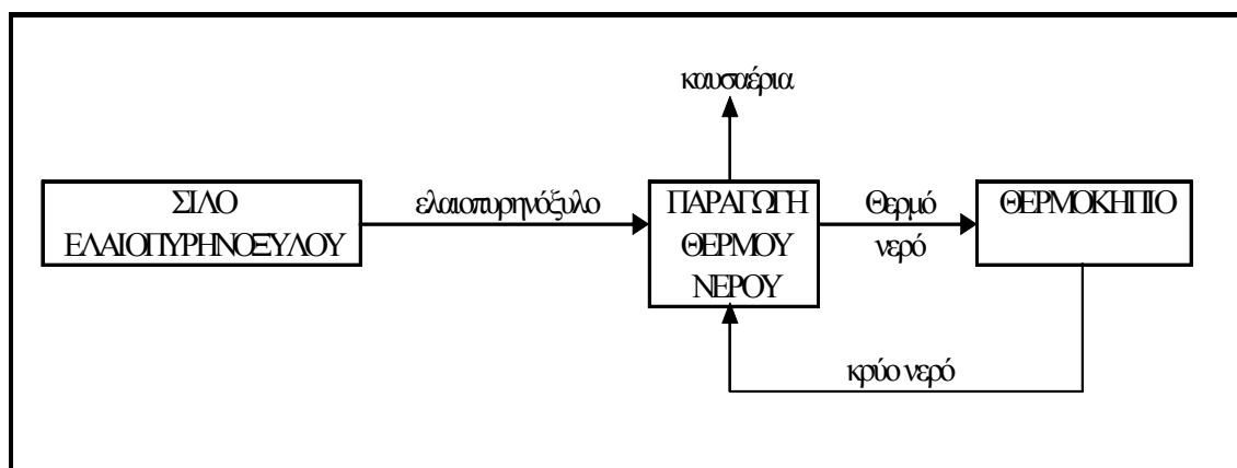
Εικόνα 46: Θέρμανση θερμοκηπίων με ελαιοπυρηνόξυλο [8]
