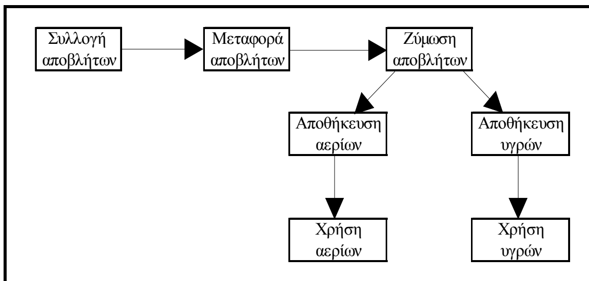
Εικόνα 12: Παραγωγή βιοαερίου από κτηνοτροφικά απόβλητα.
