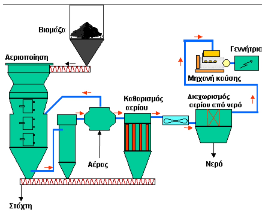
Εικόνα 11: Διεργασία καύσης βιομάζας [21]
