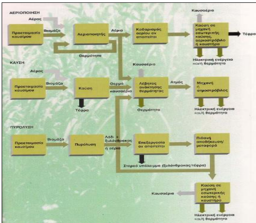
Εικόνα 44: Υπάρχουσες τεχνολογίες αξιοποίησης βιομάζας[6]
