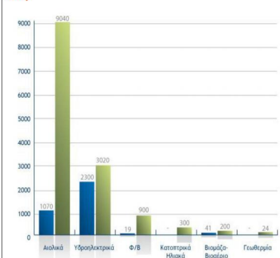
Εικόνα 43: Εξέλιξη εγκατεστημένης ισχύος ΑΠΕ [29]
