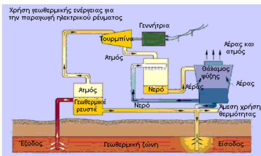
Εικόνα 5: Χρήση γεωθερμικής ενέργειας για παραγωγή ηλεκτρικού ρεύματος.[9]
