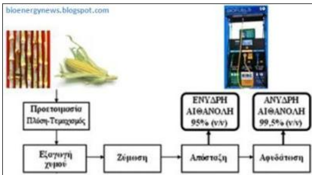
Εικόνα 13: Παραγωγή αιθανόλης από αγροτικά προϊόντα.
