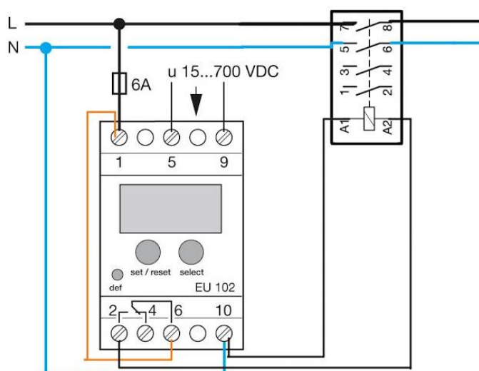
Εικόνα 1.27: 1Φ επιτηρητής και ηλεκτρονόμος στην NO επαφή. [26]
